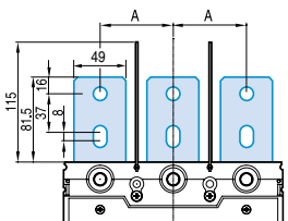
TS800 3P
