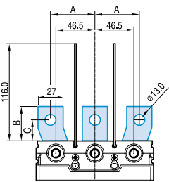
TS400, 630 3P
