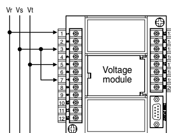
3P3W wiring
